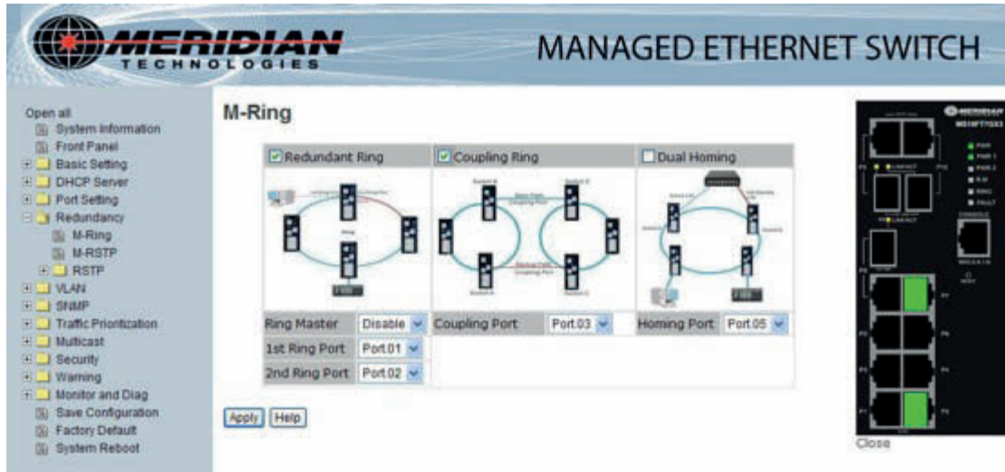
M-Ringinterface
